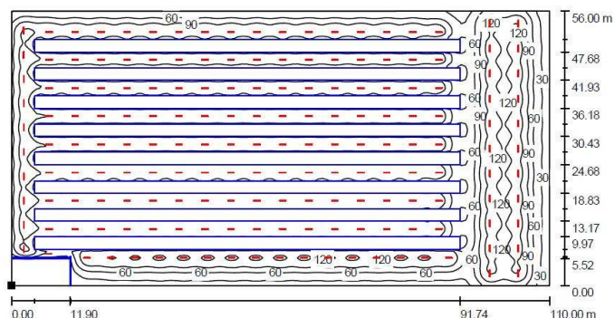
Pièce 1 / Plan utile / Courbes isolux (E)
